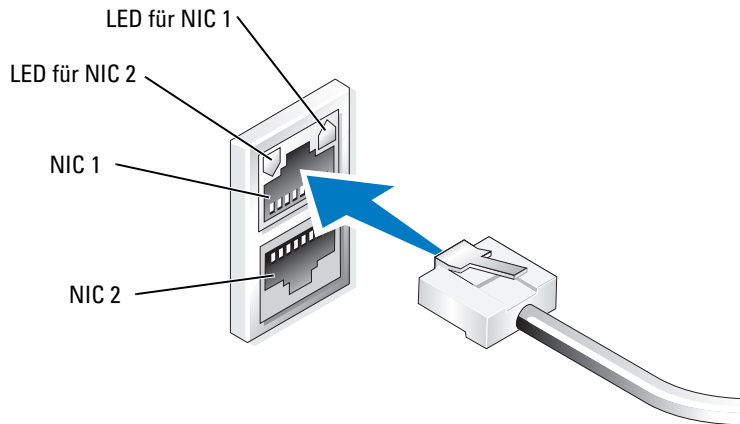
Abbildung 1-1. NIC-Anschluss
